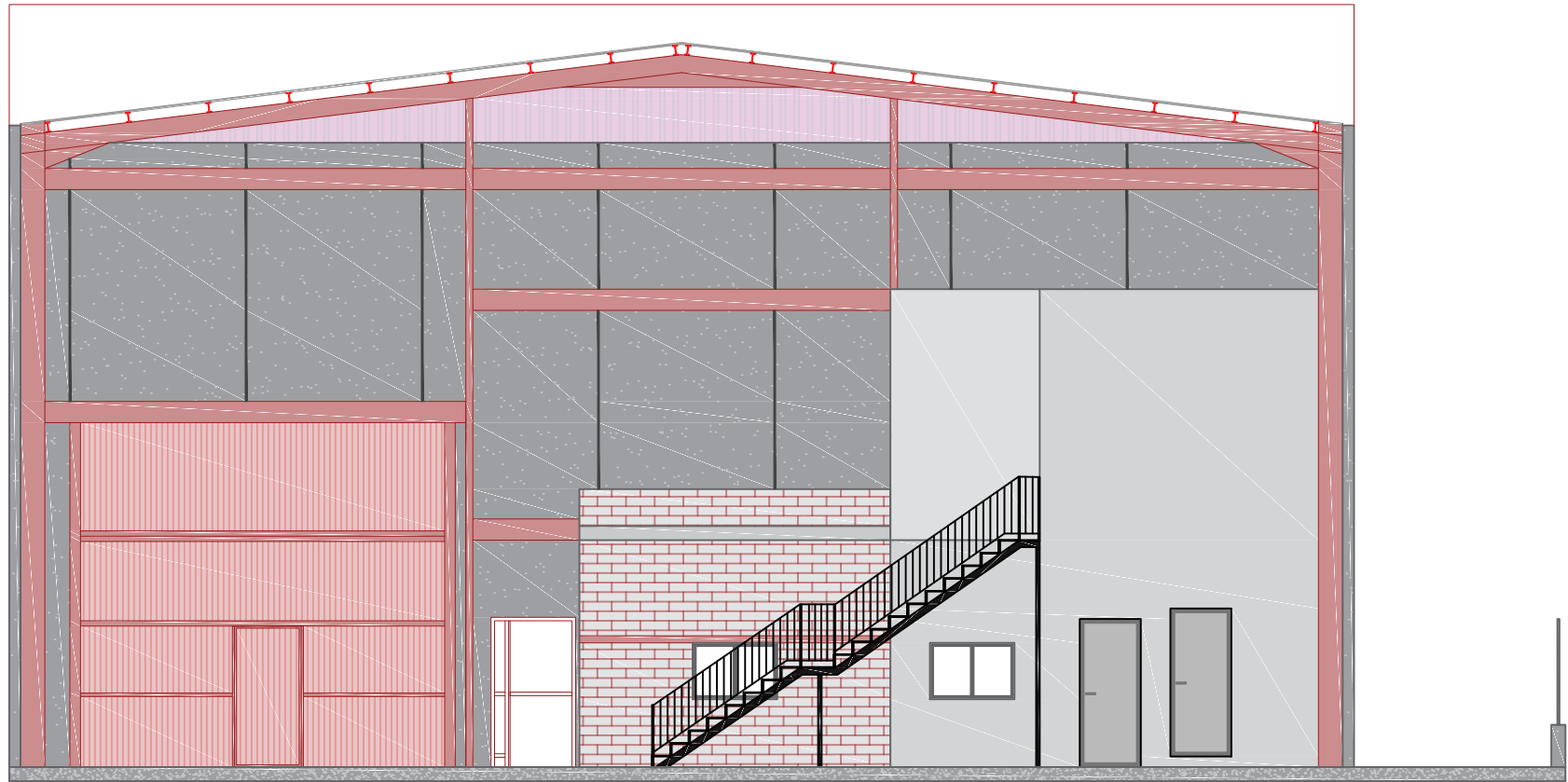
SECCIÓN A-A
