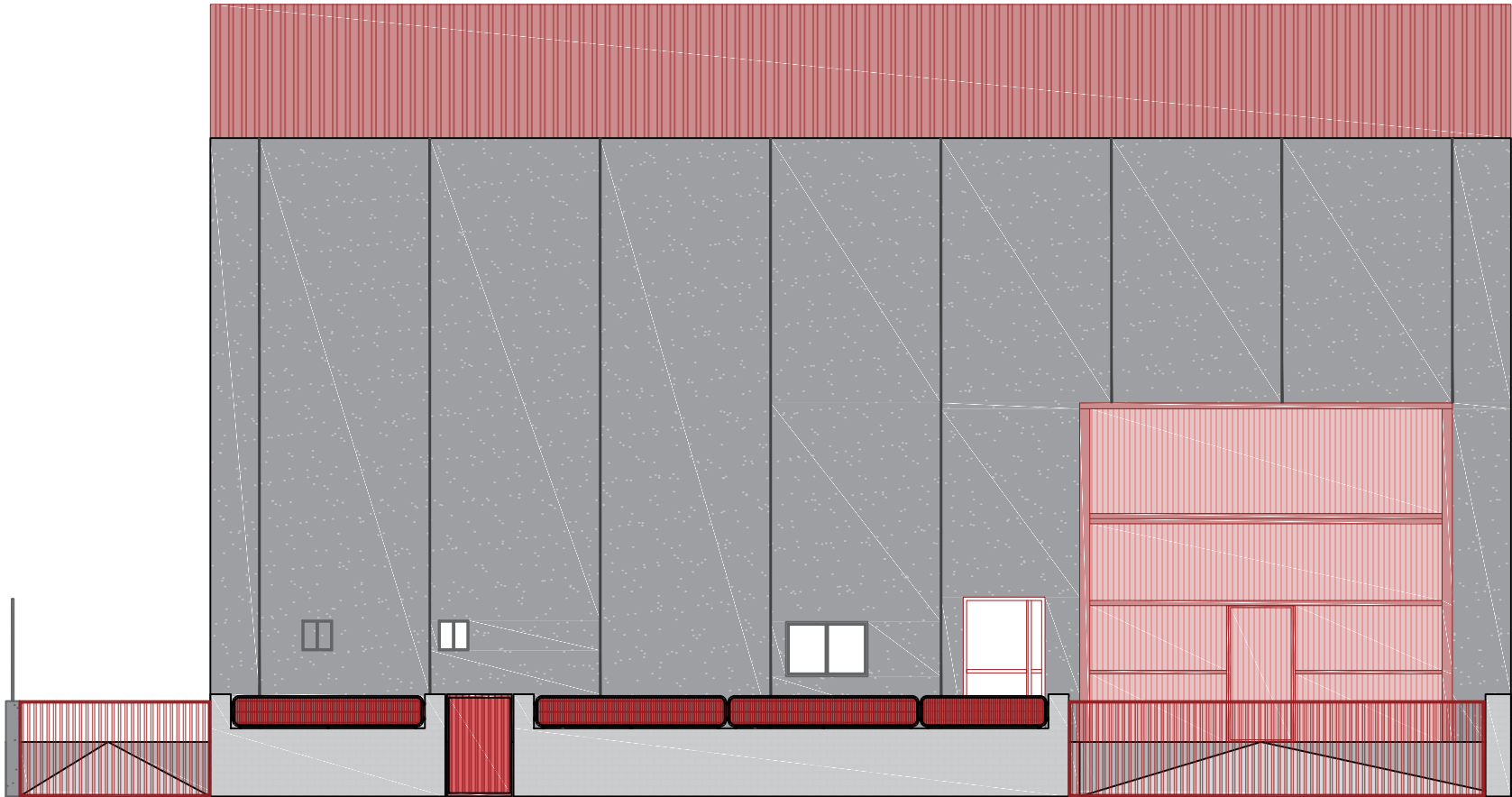
ALZADO B-B'
